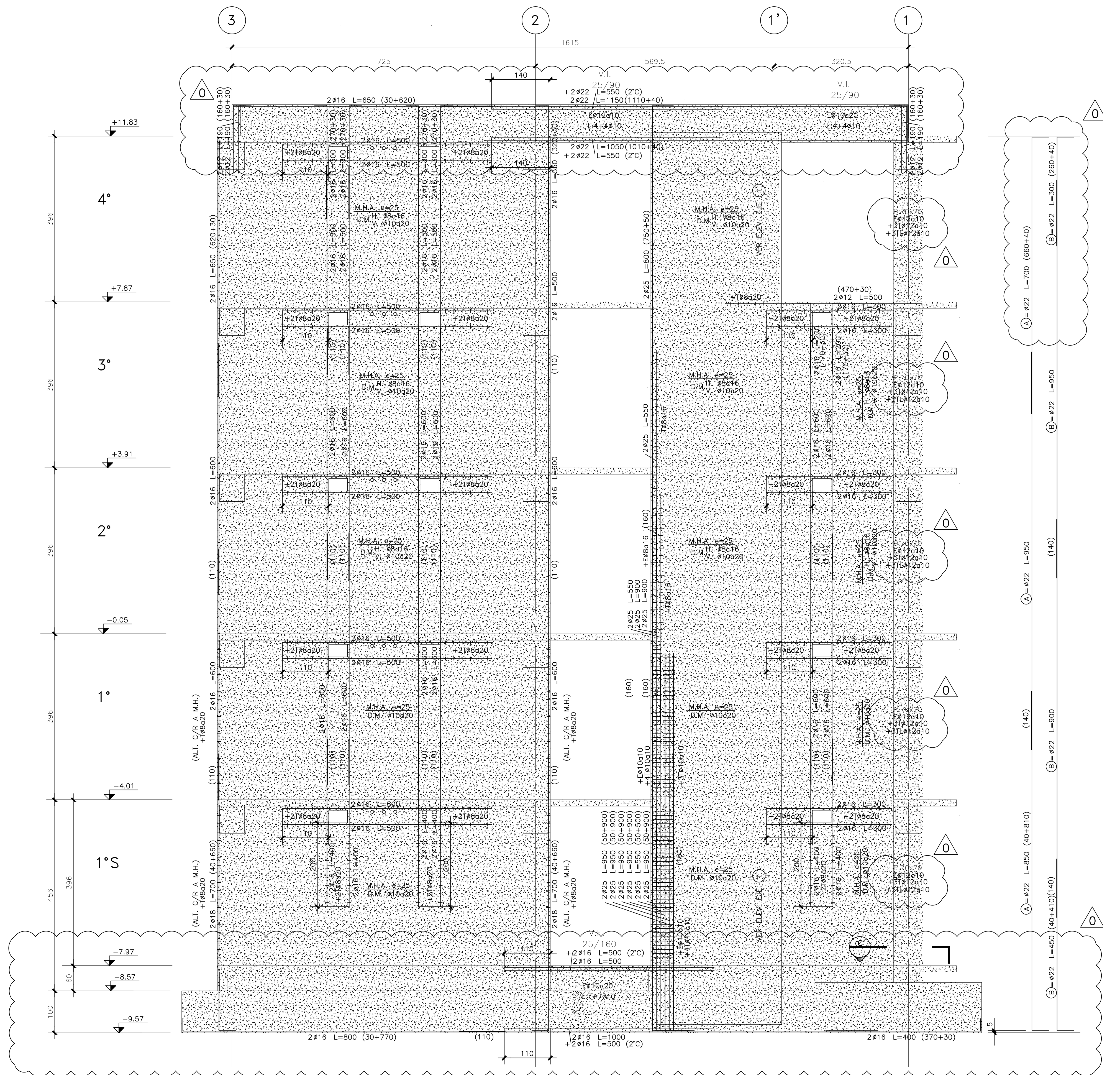
ELEVACION EJE D-D' ESCALA 1:50
