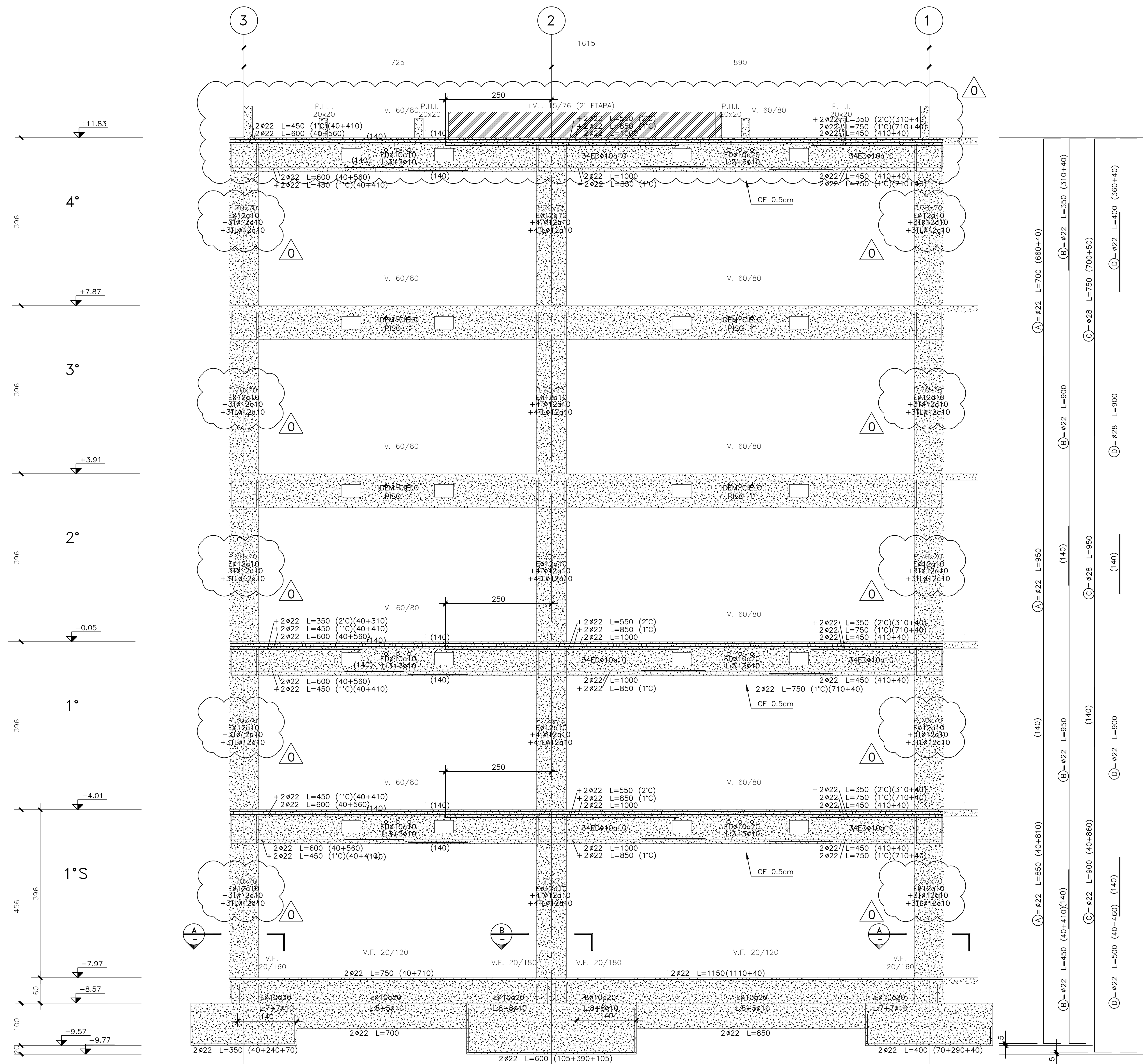
ELEVACION EJE C ESCALA 1:50
